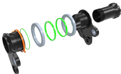
424380 SCO LINK LOWER OUTER GAMBLER 26 (sem rolamentos)
